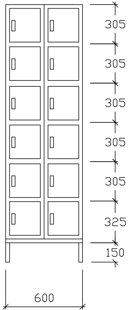
STV 60/30/2/Ug T=25(42)(52)
